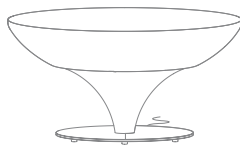
45 | Ø 845 x H450
